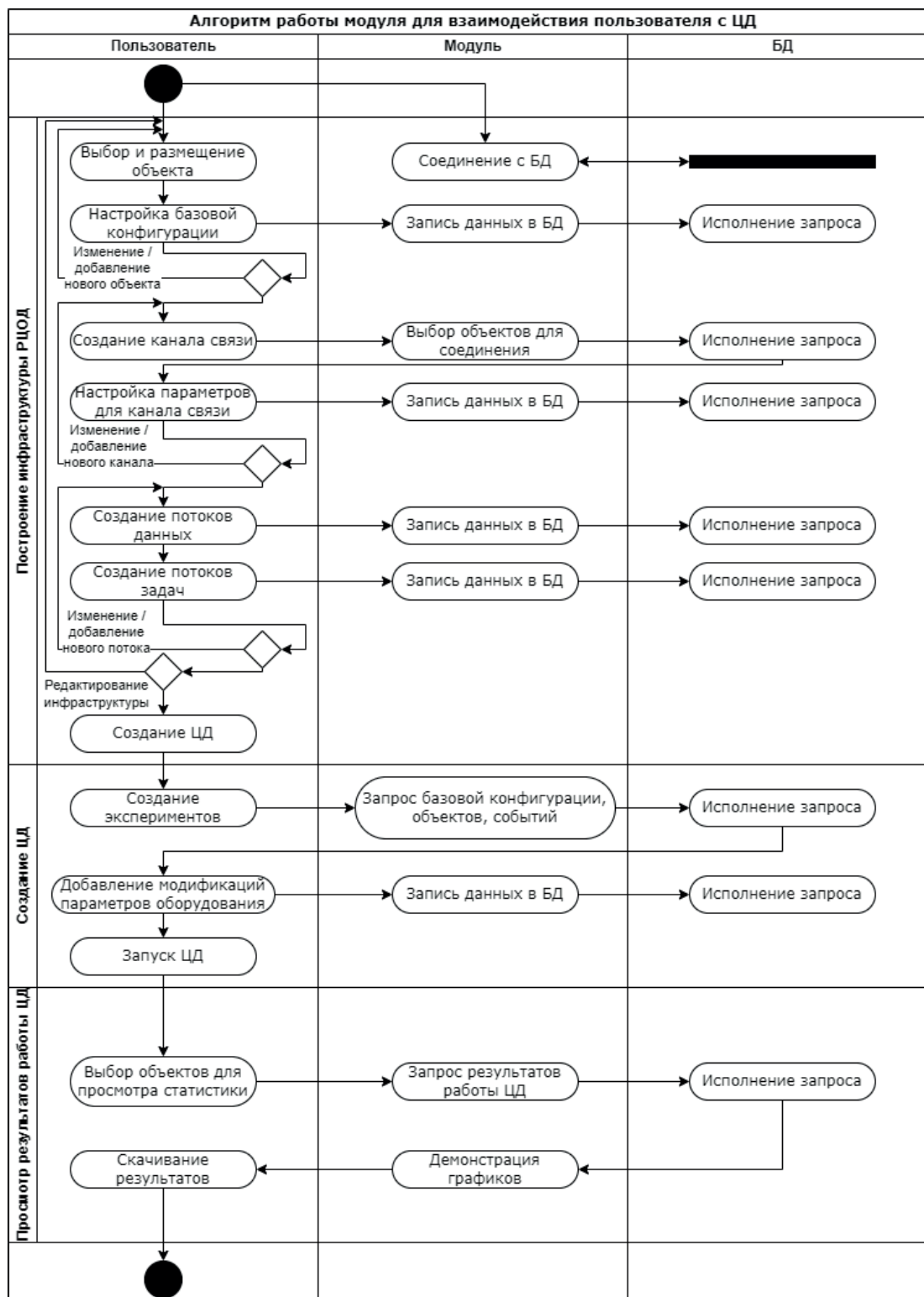
Р и с. 2. Алгоритм работы модуля для взаимодействия пользователя с цифровым двойником РЦОД
