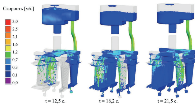
Р и с. 1. Характер заполнения керамической формы расплавленным металлом в различные моменты времени
