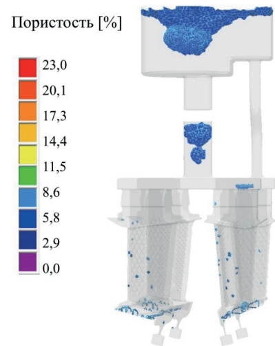
Р и с. 2. Характер распределения пористости в отливке Fig. 2. The nature of the porosity distribution in the casting
