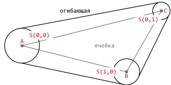
Р и с. 1. Общая огибающая множества сфер, центры которых образуют треугольник в пространстве
